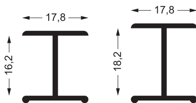
Χώρισμα Ντουλάπας "H"
