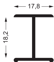
Χώρισμα Ντουλάπας "H"
