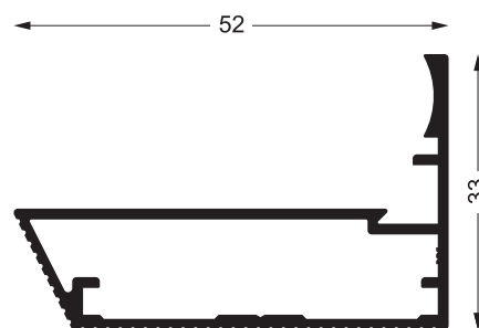
Πορτάκι P3 Χερούλι
