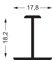
Χώρισμα Ντουλάπας H'' Slim
