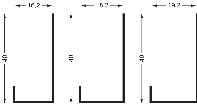
Τελείωμα Ντουλάπας "Π"
